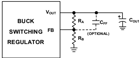
图 16. 反馈电阻网络
